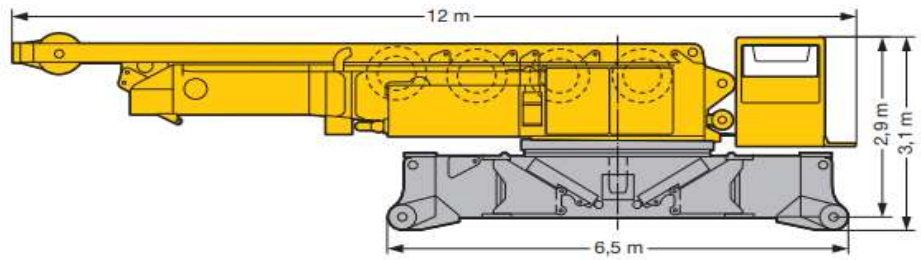
Superestructura con winche IV y Chasis central
